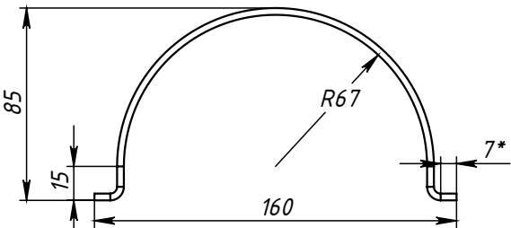
Поз.6 (Прокладка) развертка
