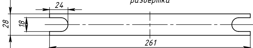
Поз.6 (Прокладка) развертка
