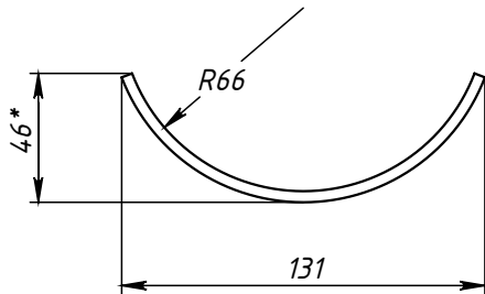
Поз.3 (Ложемент)
